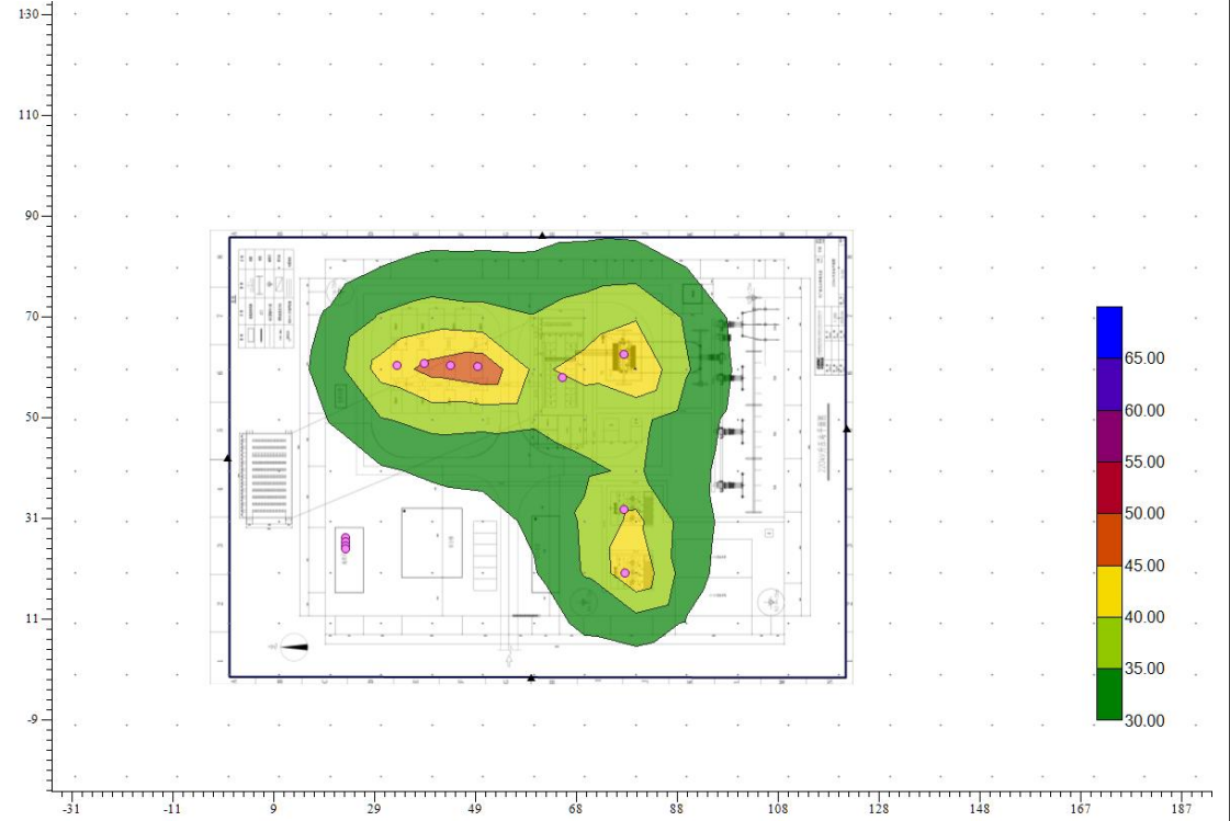
图 4-5 升压站运营期厂界噪声贡献昼间等值线图
