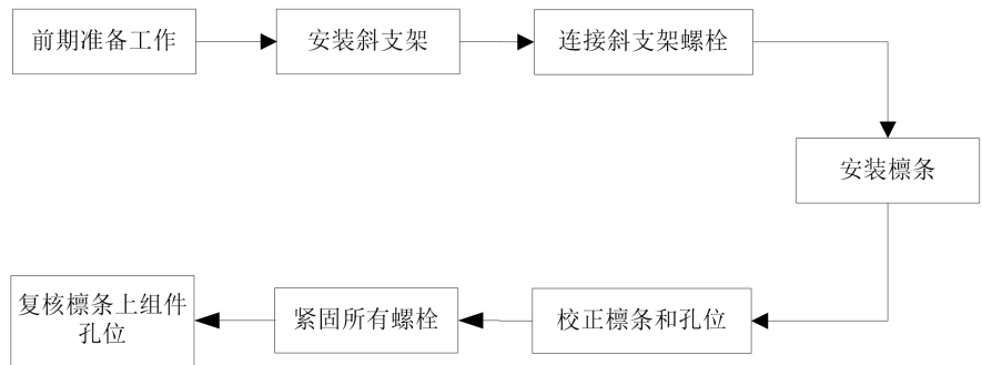
图 2-6 太阳电池组件支架安装工艺
