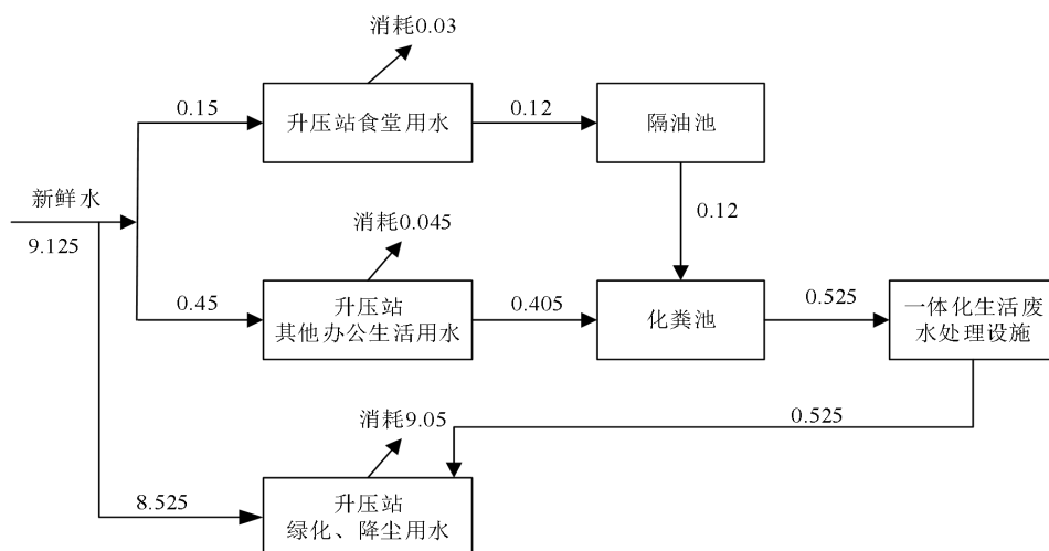
图 4-7 项目运营期间非雨天水量平衡图（未对太阳能电池板清洗时） 单位： \text{m}^3/\text{d}
