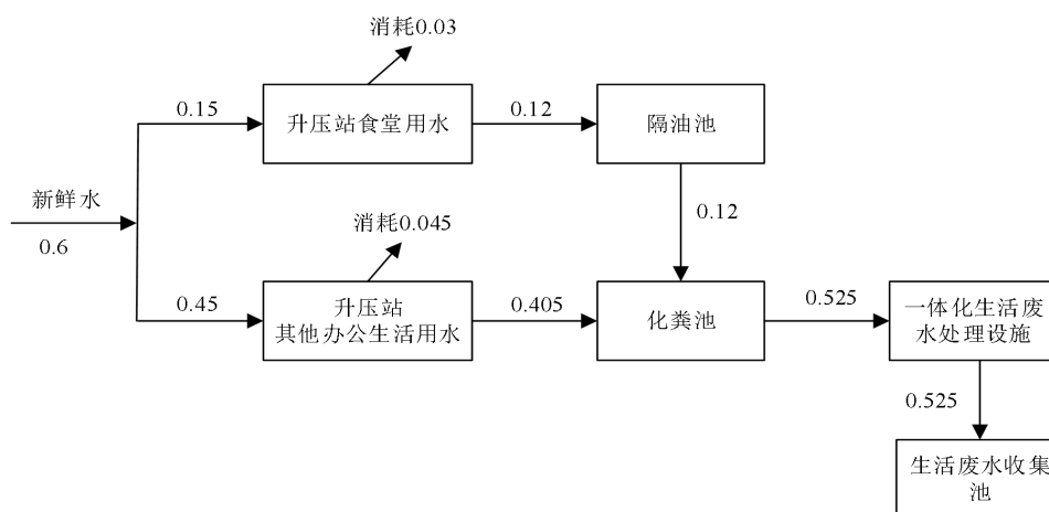
图 4-8 项目运营期间雨天水量平衡图 单位： \text{m}^3/\text{d}
