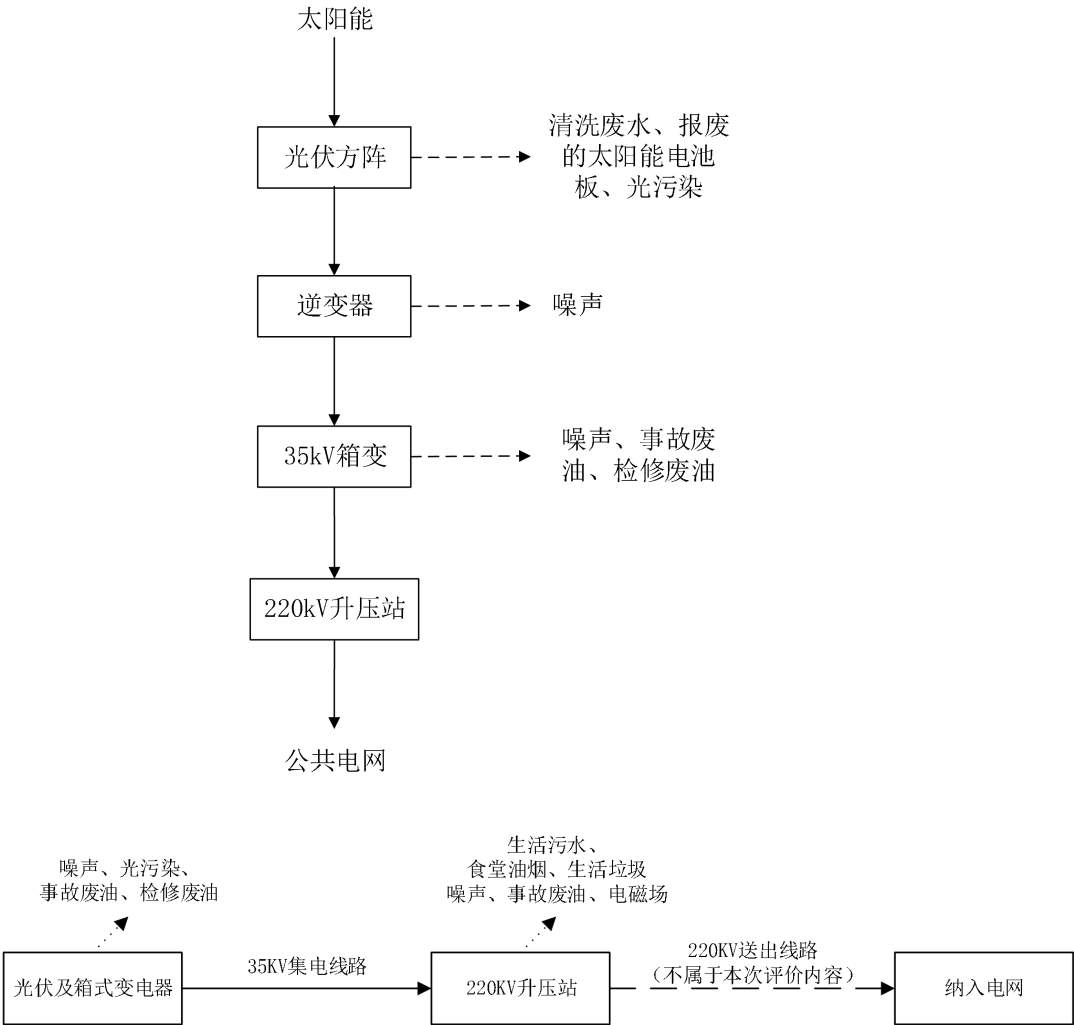
图 4-3 本项目运营期工艺流程及主要产污环节示意图
