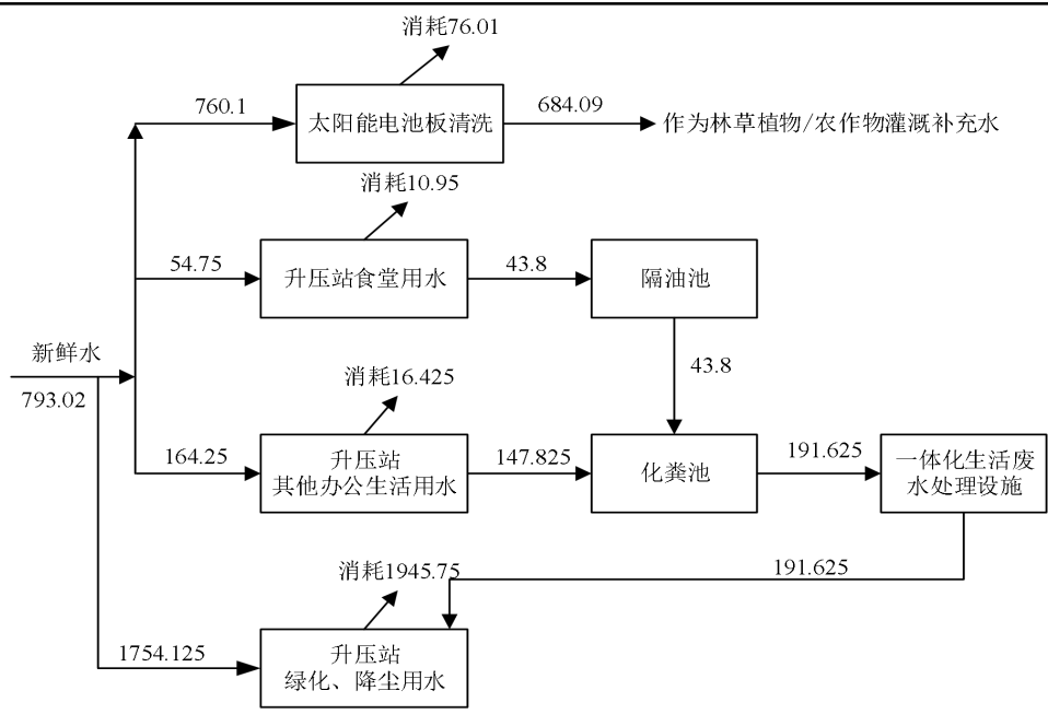
图 4-5 项目运营期全年水量平衡图 单位：m³/a
