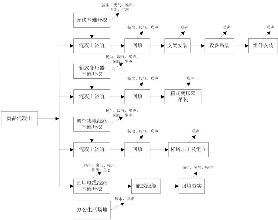
图 2-8 施工期工艺流程及产污节点
