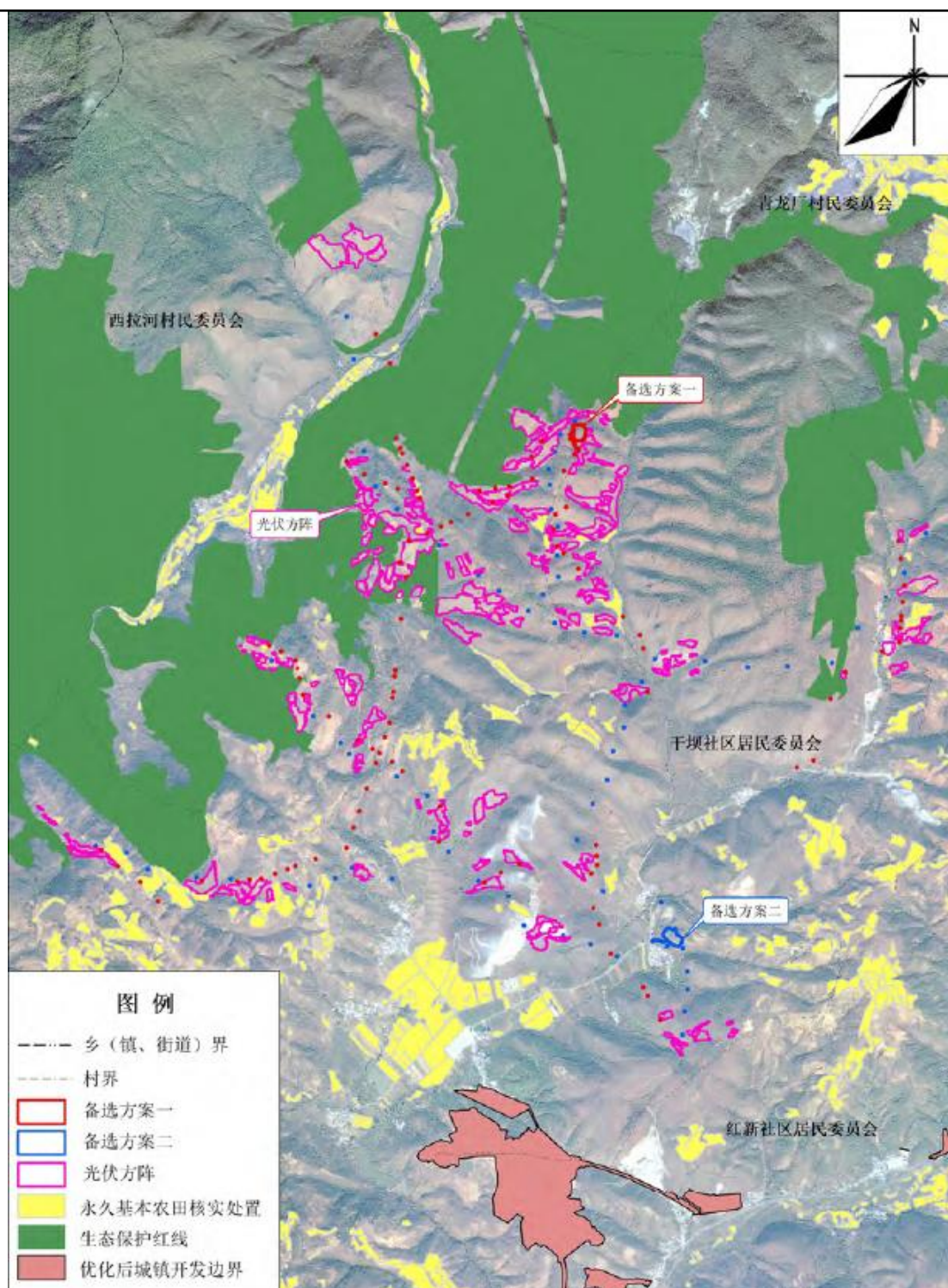
图 2-9 工程选址方案（备选方案一为项目最终实施方案）
